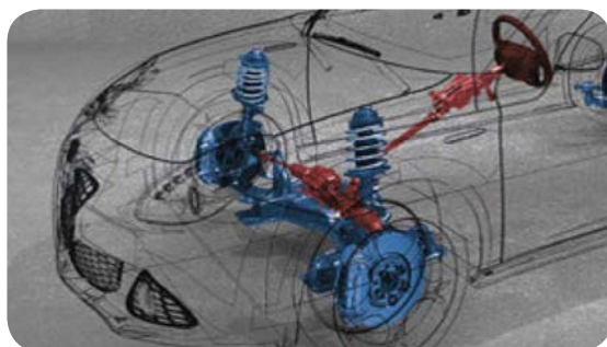
Bezpośredni układ wspomagania kierownicy
